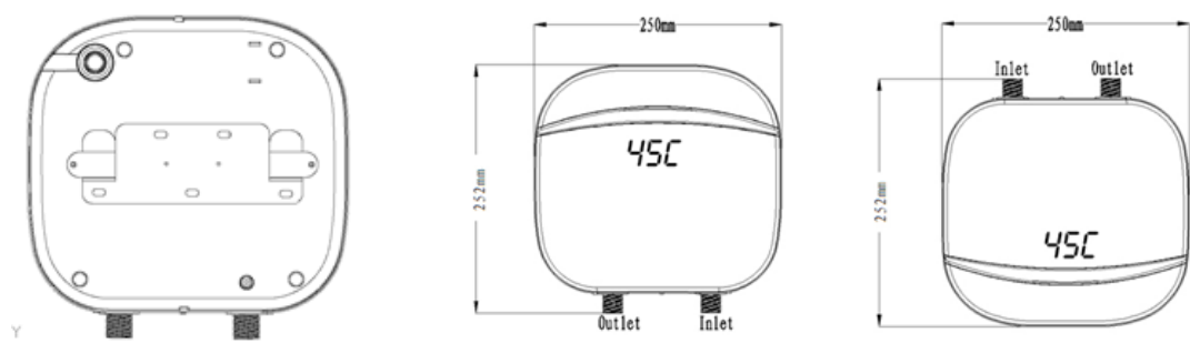
Figure 1: avant et arrière de l'appareil – installation verticale obligatoire - ne pas installer en biais (utiliser un niveau)
